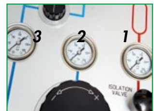
I tre manometri indicano: 1. pressione nel serbatoio 2. pressione impostata dal regolatore di pressione 3. pressione alla porta di test
